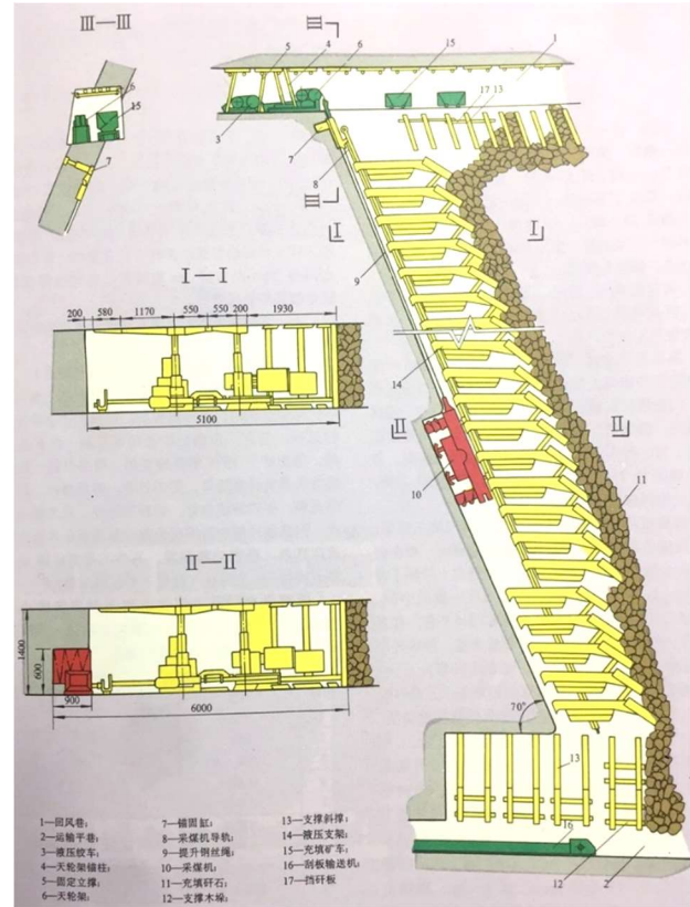
Hình 5. Sơ đồ công nghệ lò chợ khấu theo hướng xiên chéo tại một mỏ than của Trung Quốc
