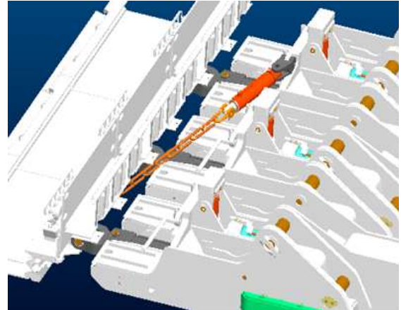
Hình 1. Giàn chống và máng cào được trang bị cơ cấu chống trôi, trượt
